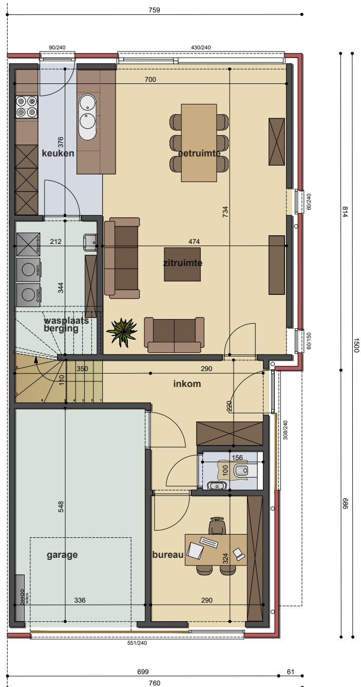
GRONDPLAN LOT 4
